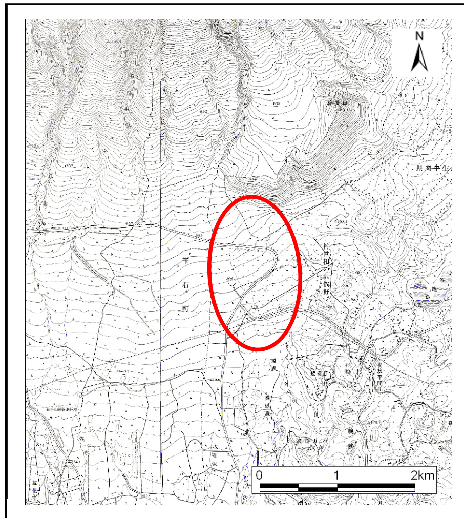
位置図(S=1:50,000)
