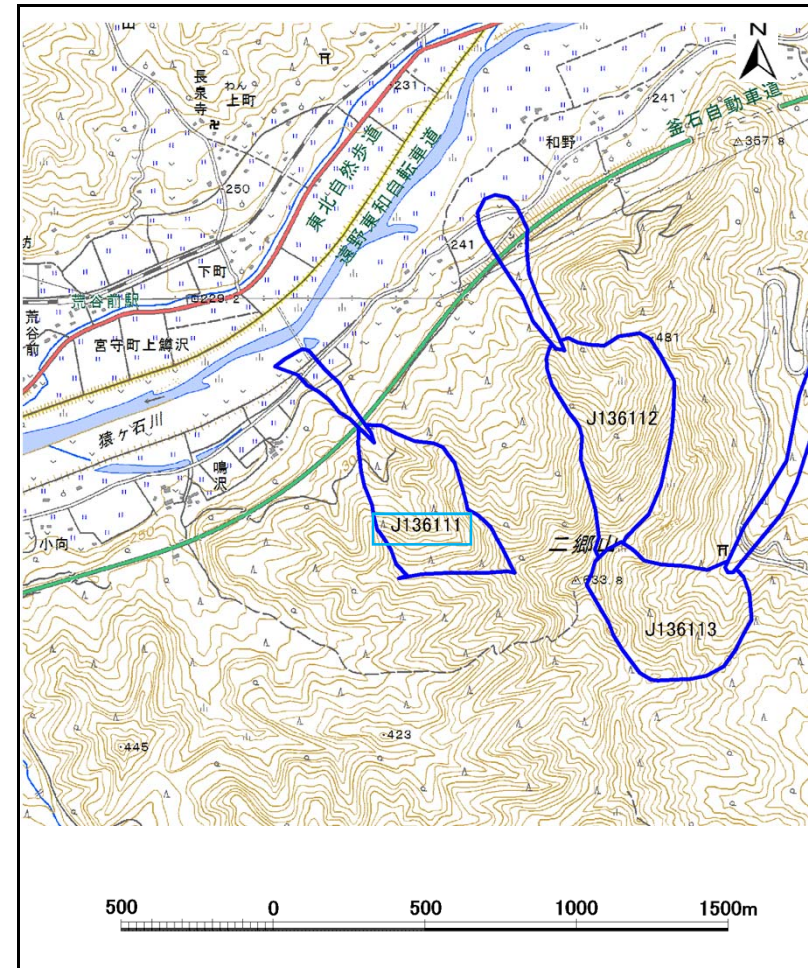
概況図(S=1:25,000)
