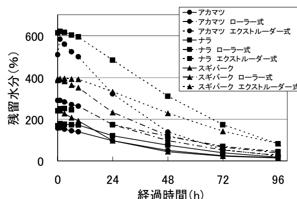
図8 残留水分の経時変化
