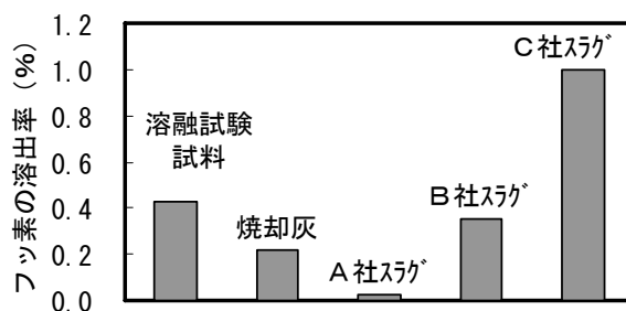
図－２ フッ素の溶出率
