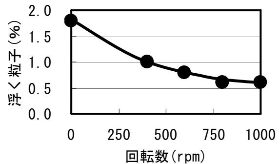
図-5 クラッシャー回転数と密度 1.95 \text{ (g/cm}^3\text{)} の液体に浮く粒子の関係
