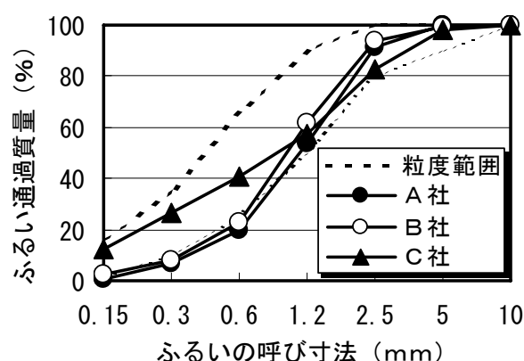
図－１ スラグ細骨材の粒度曲線
