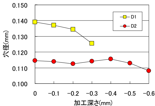
図6 Cuパイプ電極 \phi 0.1の軸穴の円筒度
