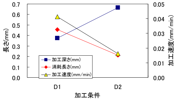
図5 Cuパイプ電極 \phi 0.1の場合
