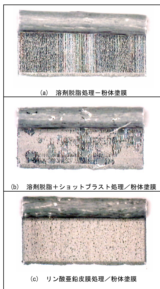
図3 粉体塗膜の切削観察写真
