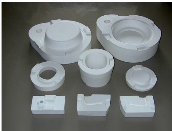
図 6 鋳込み型
