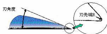
図3 鉋形状と名称
