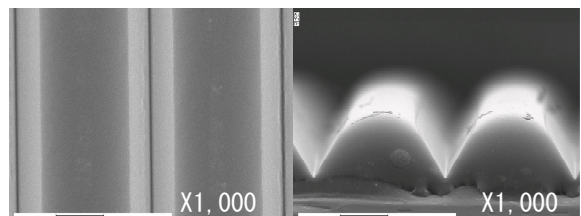
図11 電鍍金型成形品のSEM画像 (左：上から、右：横から)
