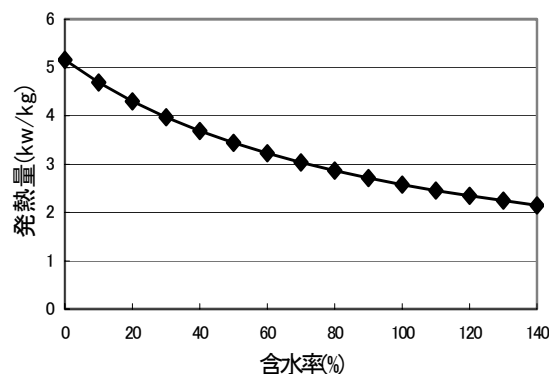
図1 含水率に対する発熱量
