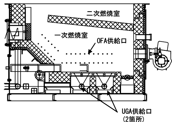
図4 燃焼室断面
