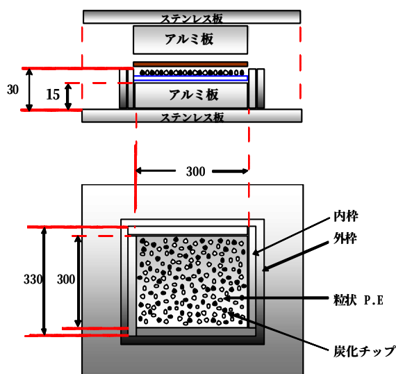
図6 成型方法
