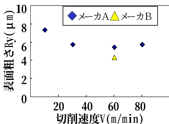
図４ 切削条件（２）における表面粗さ
