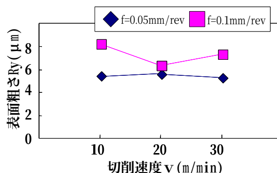
図2 切削条件(1)における表面粗さ
