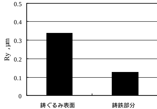
図3 鋳ぐるみ表面と鋳鉄部分の表面粗さ
