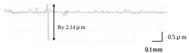
図4 鋳ぐるみ表面の粗さ曲線
