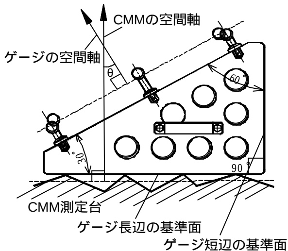
図2 反転法による直角度測定
