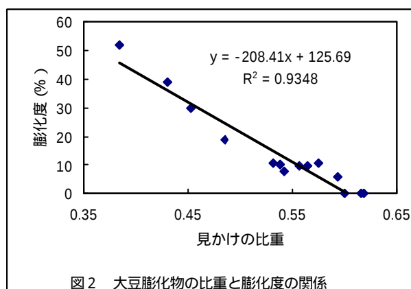
図2 大豆膨化物の比重と膨化度の関係
