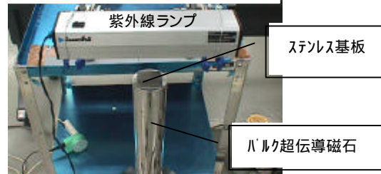
図5 バルク超伝導磁石を活用した実験の様子と磁場分布
