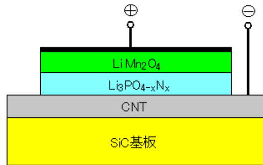
図6 CNT 薄膜を使った薄膜 Li 電池
