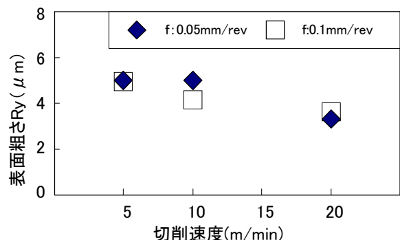
図3 加工条件変更による表面粗さ
