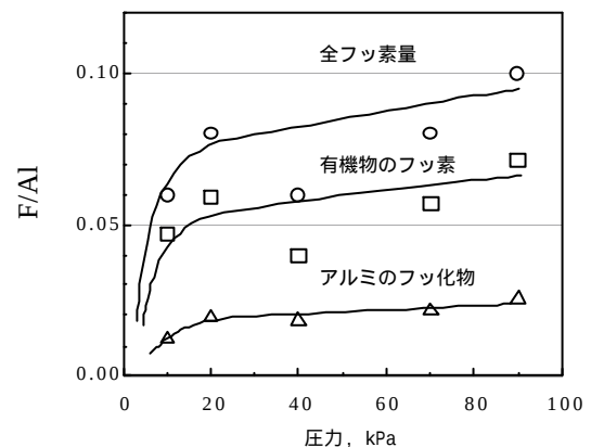
図7 圧力依存性
