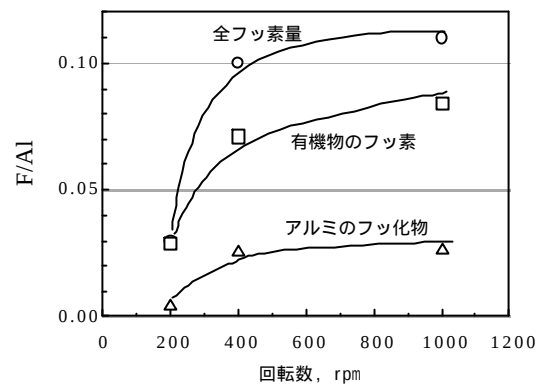
図6 回転数依存
