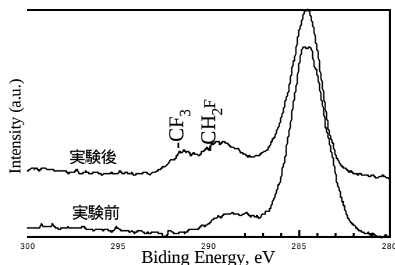
図4 C1s XPS スペクトル
