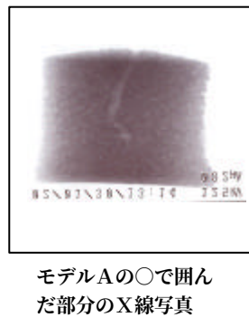
図8 OBBサンド型による鑄造試験結果
