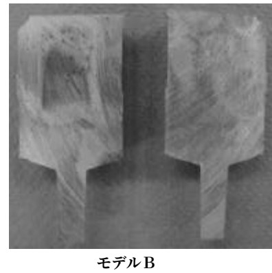
図6 引け巣危険域(色の濃い部分)
