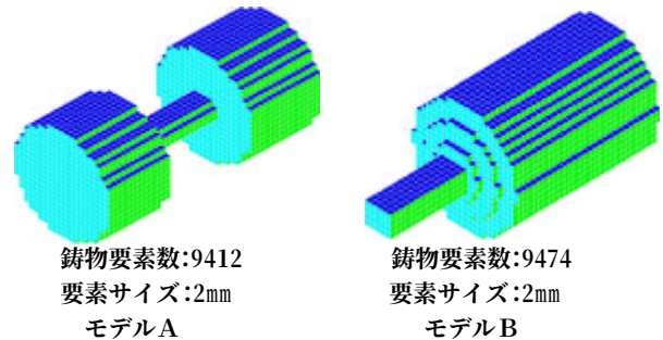
図2 解析要素
