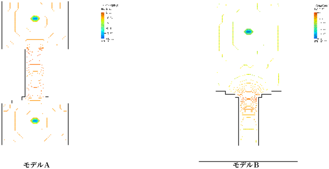
図5 G/\sqrt{R} による引け巣予測 (色の濃い部分)
