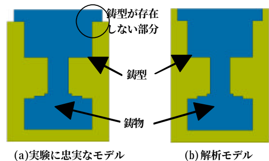
図9 実験に忠実なモデルと解析モデル
