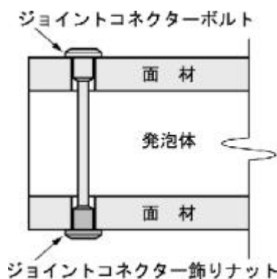
図3 金具利用のパネル構造 1
