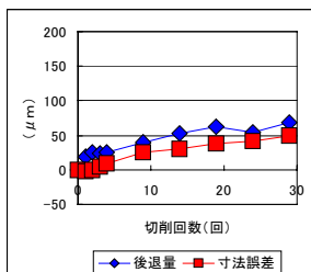
超合金 B (東芝タングロイ TH03) V100m/min, a0.2mm, f0.06mm/rev.
