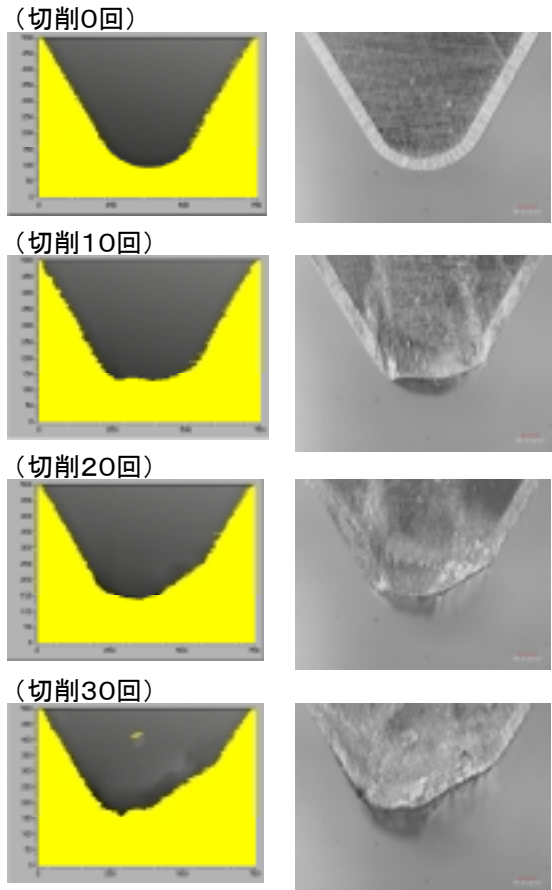
サーメットA(京セラN) v300m/min,a0.2mm,f0.06mm/rev.
