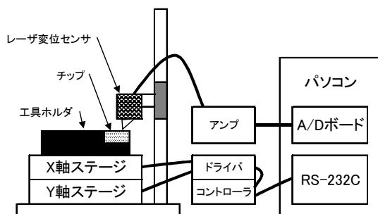
図1 測定装置構成図
