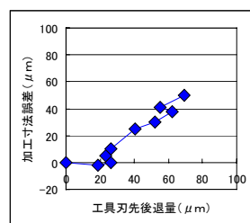
超合金 B (東芝タングロイ TH03) V100m/min, a0.2mm, f0.06mm/rev.
