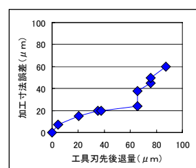
超合金 A (京セラ KW-10) V100m/min, a0.2mm, f0.06mm/rev.
