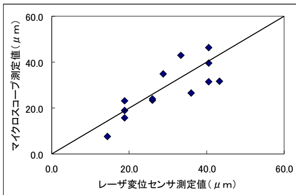
図3 レーザ変位センサ計測誤差
