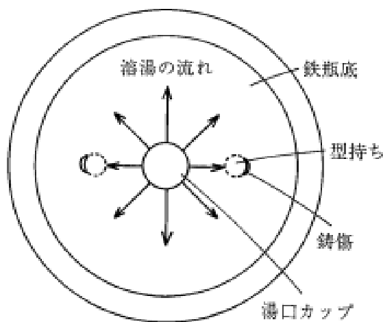
図2 鉄瓶底の鋳傷発生形態
