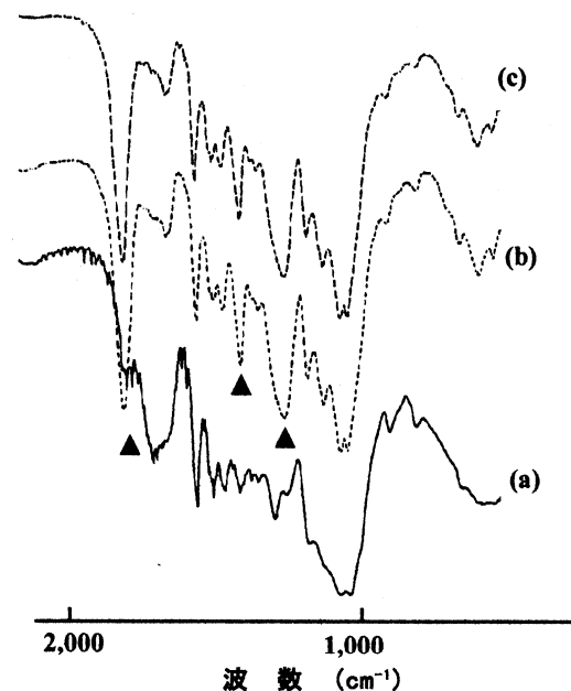
図3 合成温泉水処理されたスギのFT-IRスペクトル アセチル化条件: 110℃, 2h.
