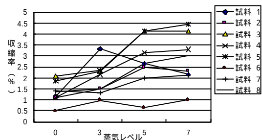
図8 120における蒸気レベルと収縮率の関係
