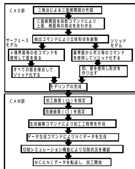
図2 3次元CAD/CAMの操作の流れ
