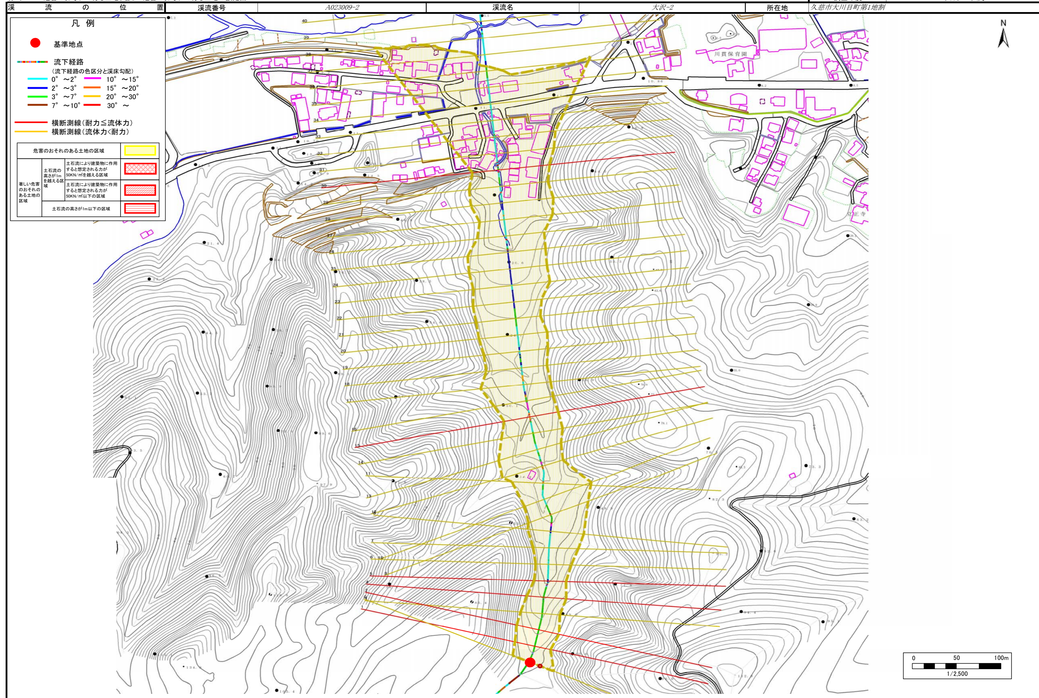
様式3-1 危険のおそれのある土地、著しい危険のおそれのある土地の設定図
