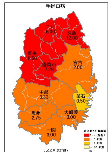
図2 第37週の保健所管内別の状況
