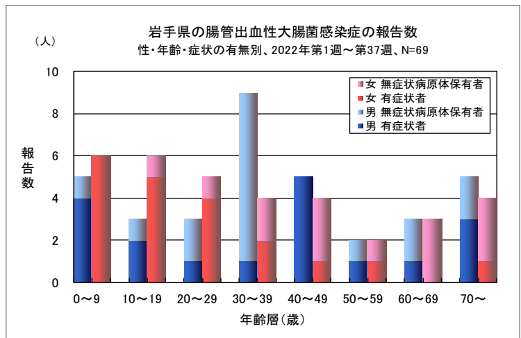
図4 岩手県の年齢性別発生状況 (2022年第1週～第37週)
