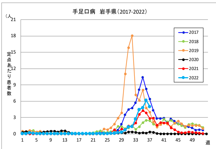
図1 岩手県における週別患者報告数 (2017年～2022年第37週)
