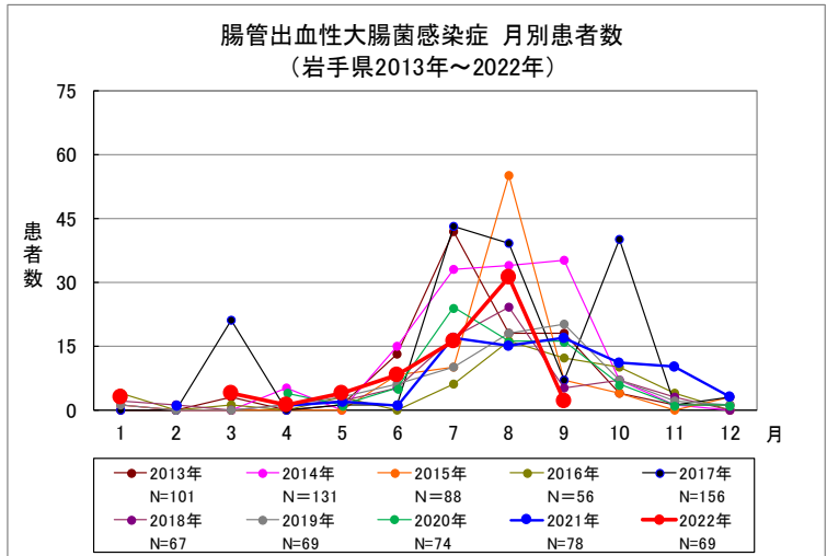
図2 岩手県の過去10年の月別発生状況 (2013年～2022年第37週)
