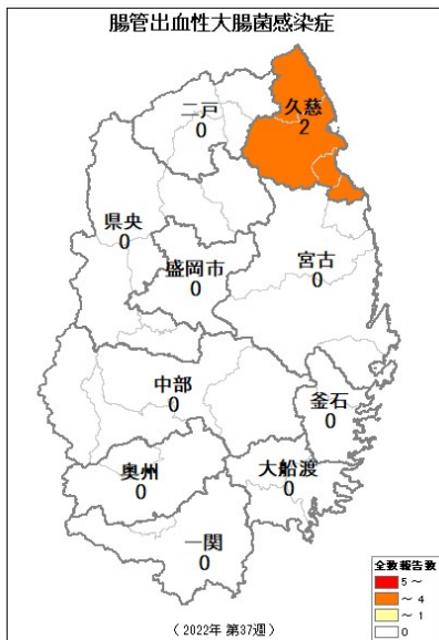
図3 第37週の保健所管内別の状況
