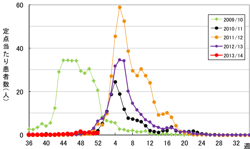
インフルエンザ、岩手県 (2009/10-2013/14)
