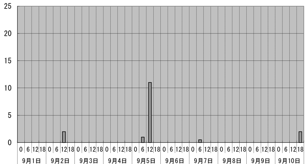
降水量mm
