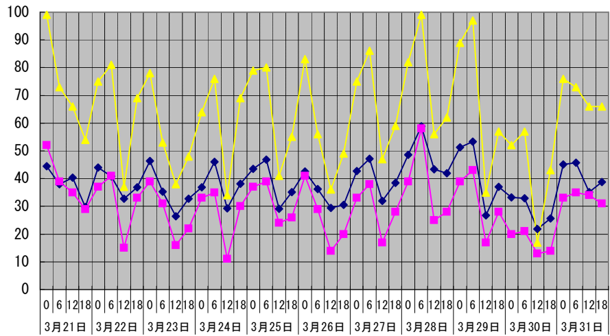
湿度%
