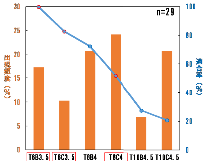
図 乾燥スケジュールごとの出現頻度と適合率(エンジュ)
