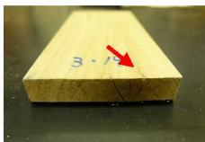
写真2 初期割れ
