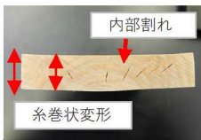
写真3 試験体断面
