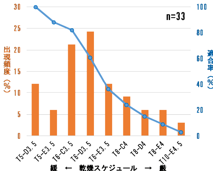
図 乾燥スケジュールごとの出現頻度と適合率(オニグルミ)
