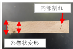
写真3 内部割れ、糸巻状変形
