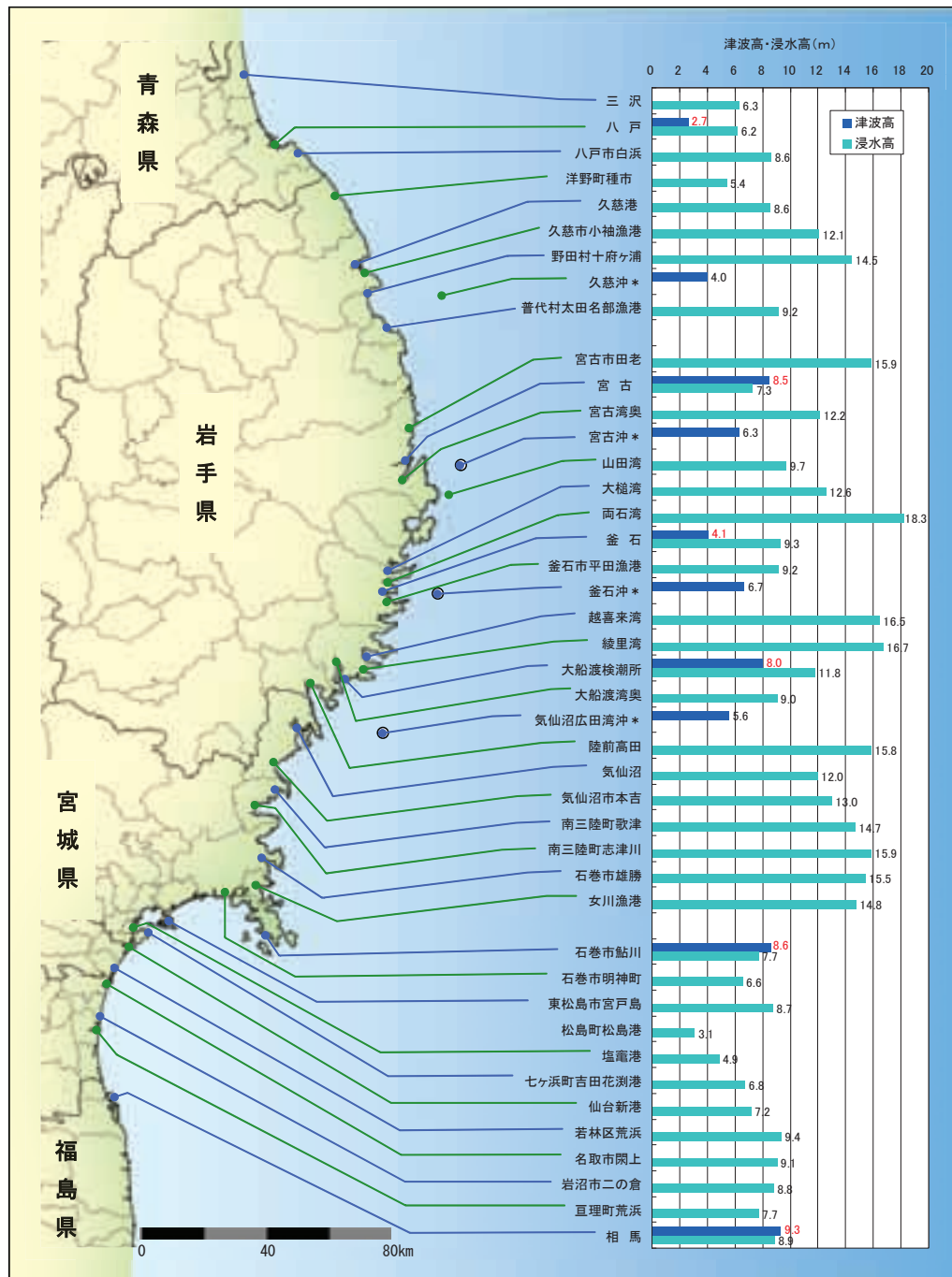
図1-7 各地の津波高・浸水高
