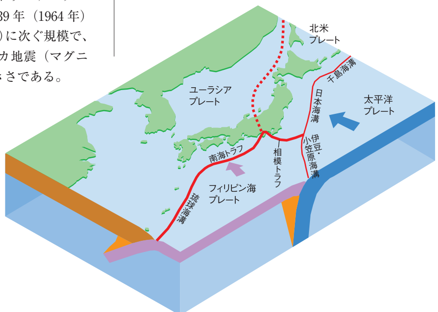
図1-1 日本付近のプレート
