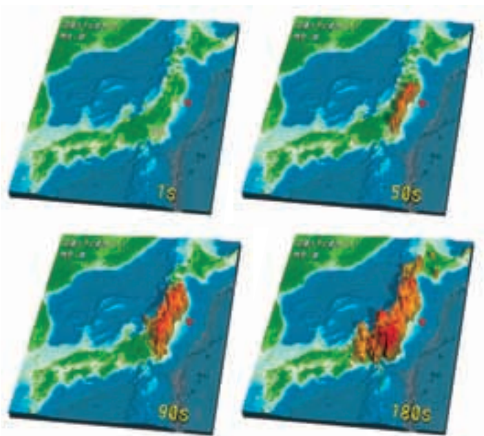
図1-4 揺れの広がる様子
