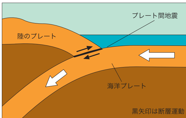
図1-2 プレート間地震
